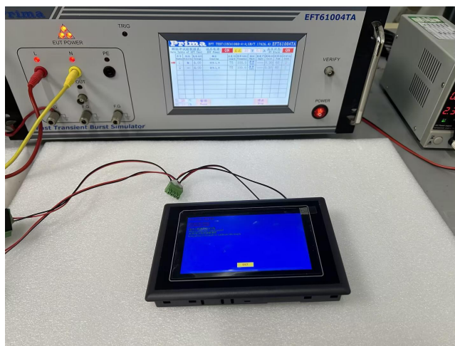
图 5-3 EFT 测试图
