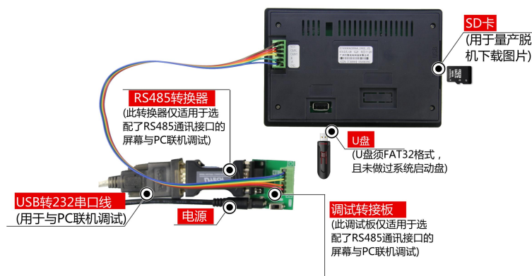
图 1-3 RS485 调试工具图
